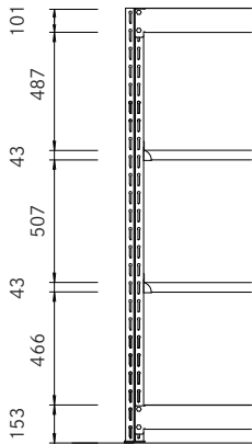
1800H 天地4段
