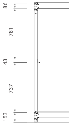
1800H 天地3段
