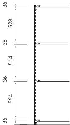
1800H 天地4段
