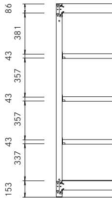
1800H 天地5段
