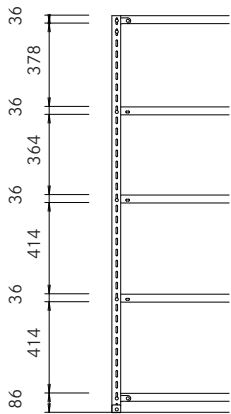
1800H 天地5段
