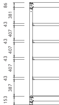
棚段増価格
