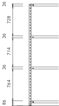
2400H 天地4段
