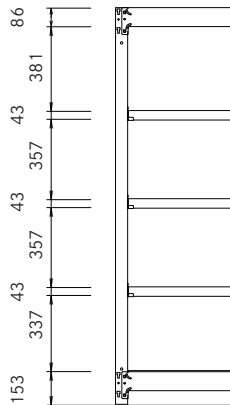
1800H 天地5段
