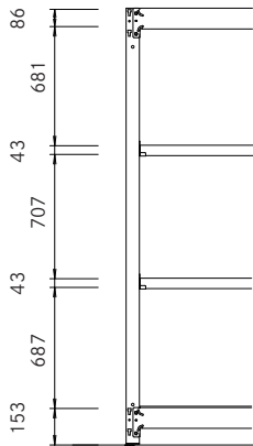
2400H 天地4段
