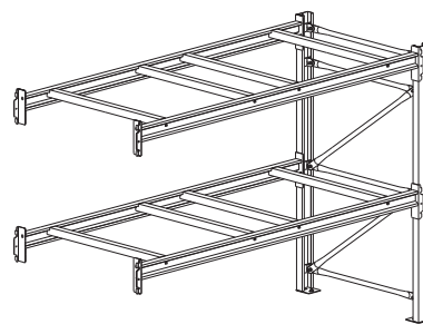
連結
