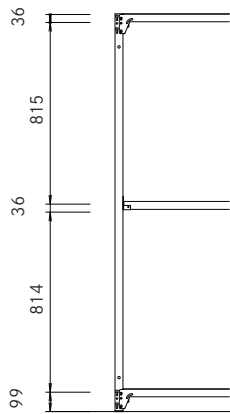
1800H 天地3段
