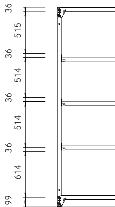
2400H 天地5段
