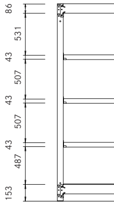
2400H 天地5段
