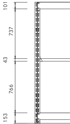
1800H 天地3段
