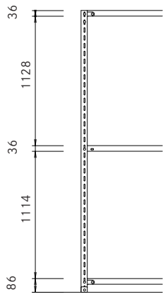
2400H 天地3段
