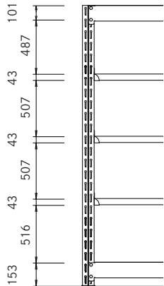
2400H 天地5段
