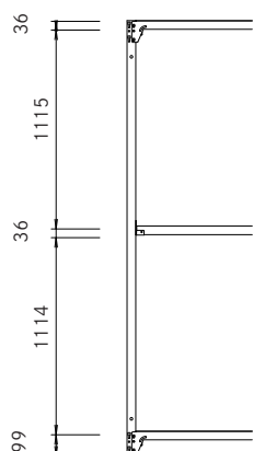
2400H 天地3段
