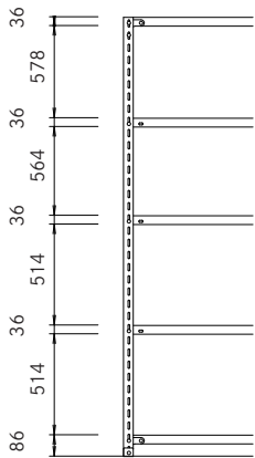
2400H 天地5段
